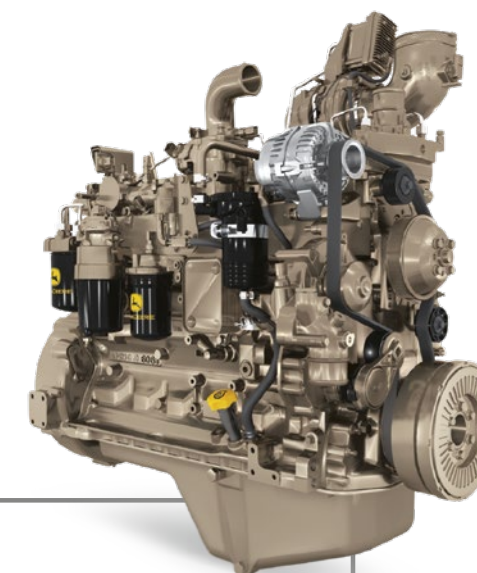
Motore PSS da 6,8 l
